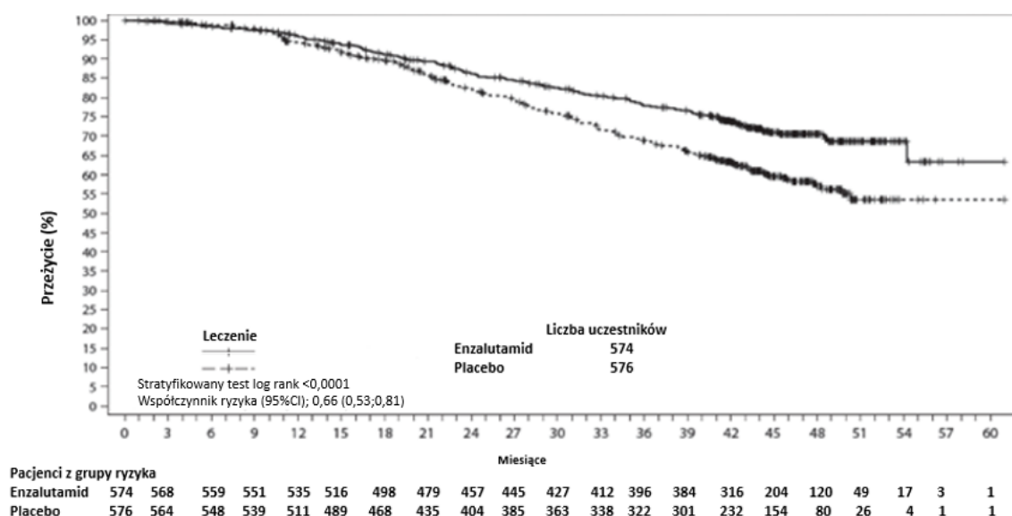
Rycina 4: Krzywe Kaplana-Meiera dotyczące całkowitego czasu przeżycia w badaniu ARCHES (analiza populacji zgodnej z zaplanowanym leczeniem)
